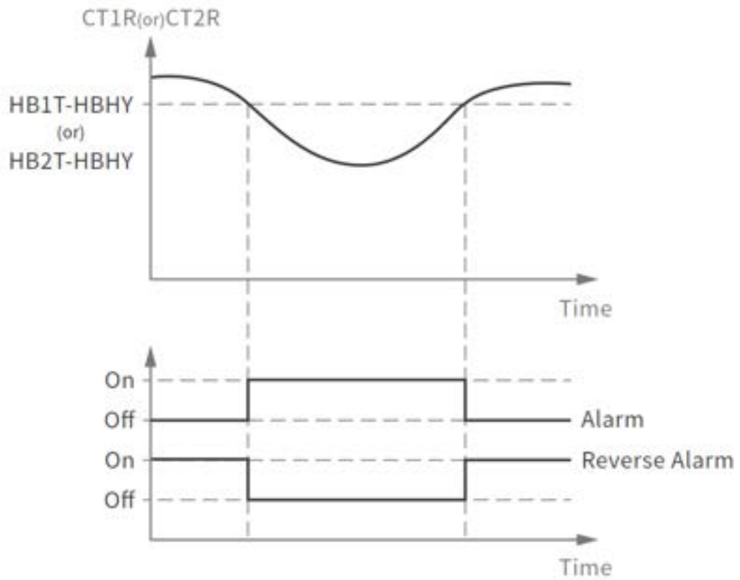
3-11 Heater Break(H.bk)
