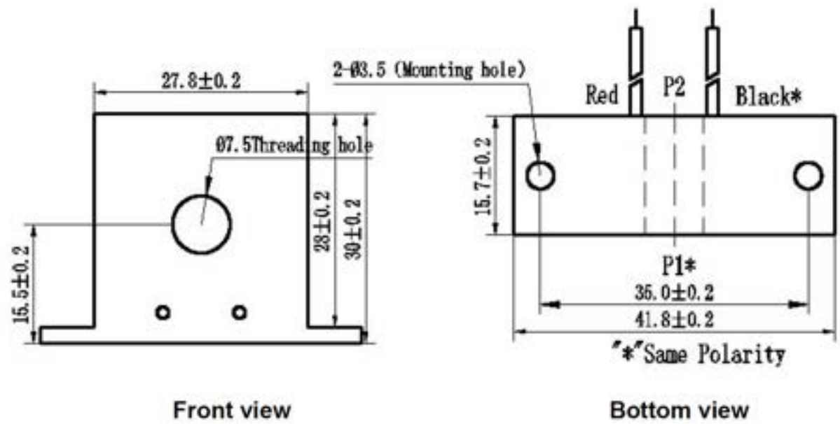
2-14 CT98-1 Dimension
