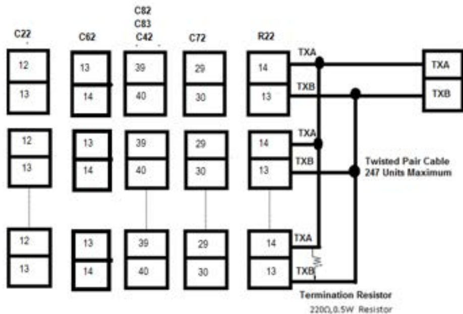
2-42 RS-485 Wiring
